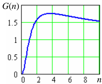
Рис. 4. Изменение аттрактора для среднегеометрического
