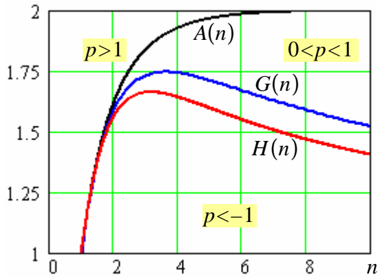
Рис. 5. Изменение степенных аттракторов
